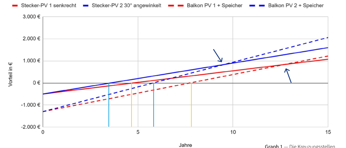
Graph 1 — Die Kreuzungsstellen markieren den Zeitpunkt, ab dem durch das Steckersolargerät mit Speicher mehr Geld gespart wird, als ohne •
