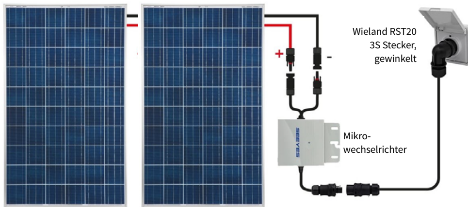
Abb 2 — Beispielhafter Aufbau einer steckerfertigen Solaranlage. Foto: greenakku.de / Bosswerk GmbH & Co. KG •
