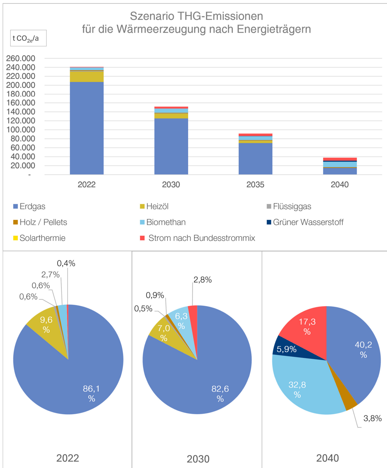
Abbildung 26: Zielszenario THG-Emissionen nach Energieträgern bis 2040 (Quelle: Analyseergebnisse OCF Consulting)
