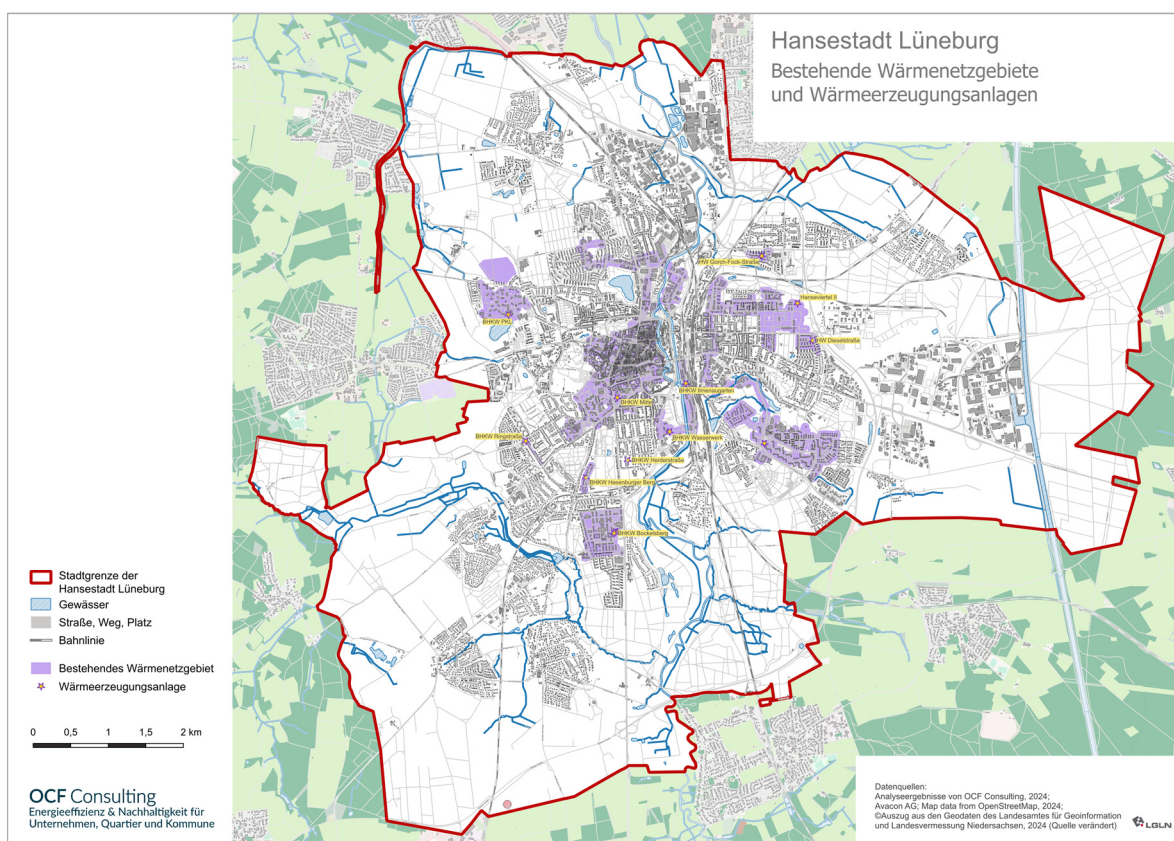
Abbildung 17: Wärmenetze und Wärmeerzeugungsanlagen in der Übersicht (Quelle: OCF Consulting)
