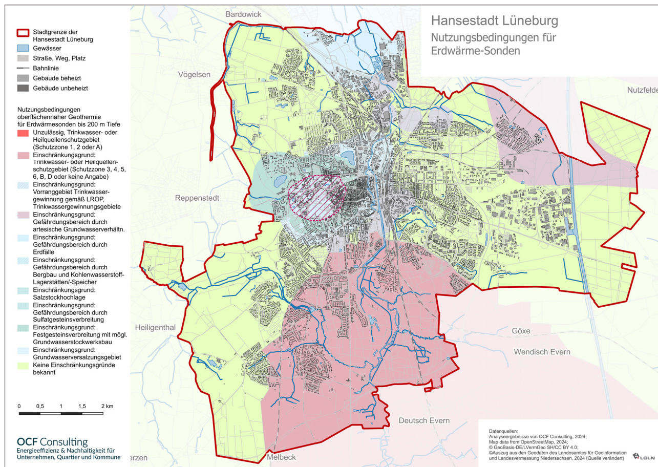
Abbildung 22: Nutzungsbedingungen oberflächennaher Geothermie für Erdwärmesonden (bis 200 m Tiefe) (Quelle: OCF Consulting basierend auf Daten des LBEG)
