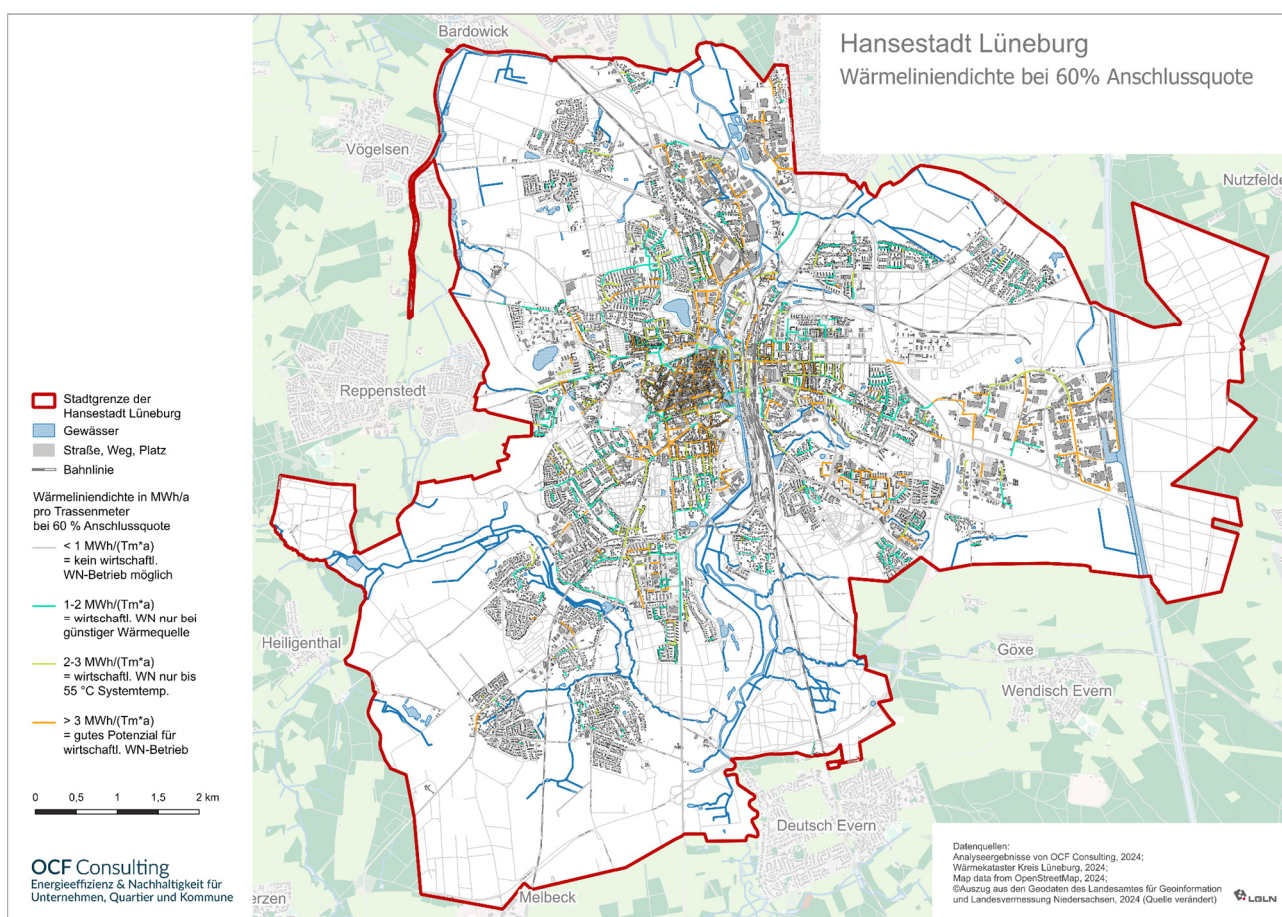
Abbildung 13: Wärmeliniendichte Lüneburg für das Jahr 2022 in MWh pro Tm und Jahr bei 60 % Anschlussquote an ein fiktives Wärmenetz (WN) (Quelle: OCF Consulting auf Basis des Wärmekatasters Kreis Lüneburg)
