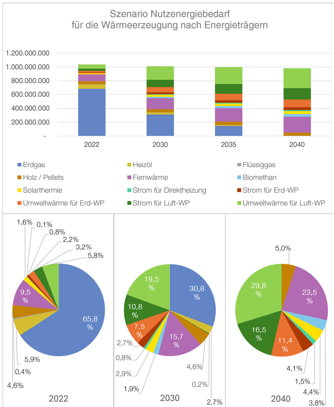
Abbildung 24: Zielszenario – Wärmebedarf (Nutzenergiebedarf) nach Energieträgern bis 2040 (Quelle: Analyseergebnisse OCF Consulting)
