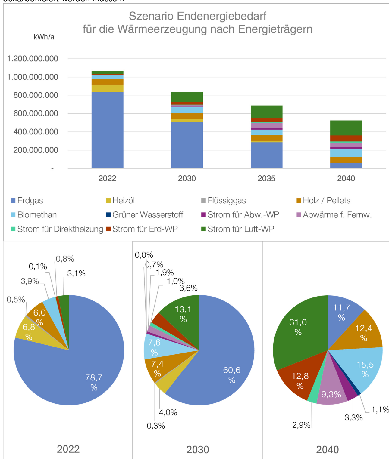
Abbildung 25: Zielszenario Endenergiebedarf nach Energieträgern bis 2040 (Quelle: Analyseergebnisse OCF Consulting)
