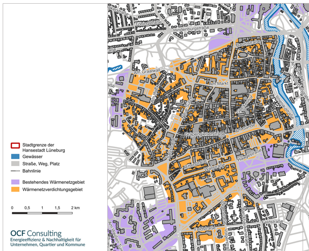
Abbildung 27: Wärmenetzverdichtungsgebiet innerhalb des Bestandwärmenetzes Mitte (violett) mit Nachverdichtungspotenzial (orange) (Quelle: OCF Consulting)
