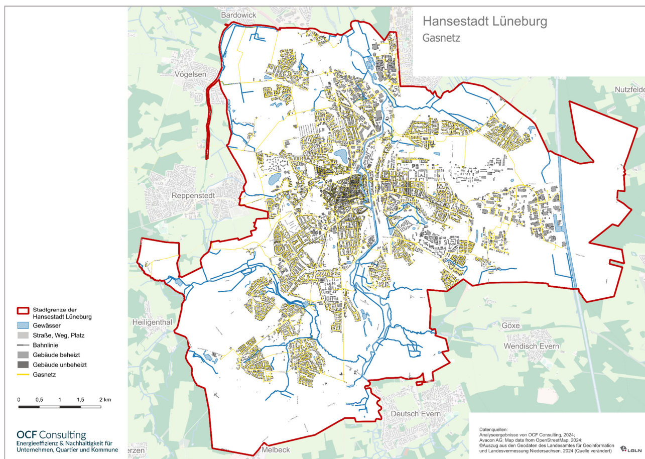
Abbildung 15: Gasnetz in Lüneburg (Quelle: OCF Consulting)
