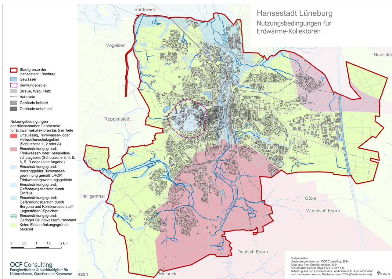
Abbildung 23: Nutzungsbedingungen für Erdwärmekollektoren bis zu 5 m Tiefe (Quelle: OCF Consulting basierend auf Daten des LBEG)
