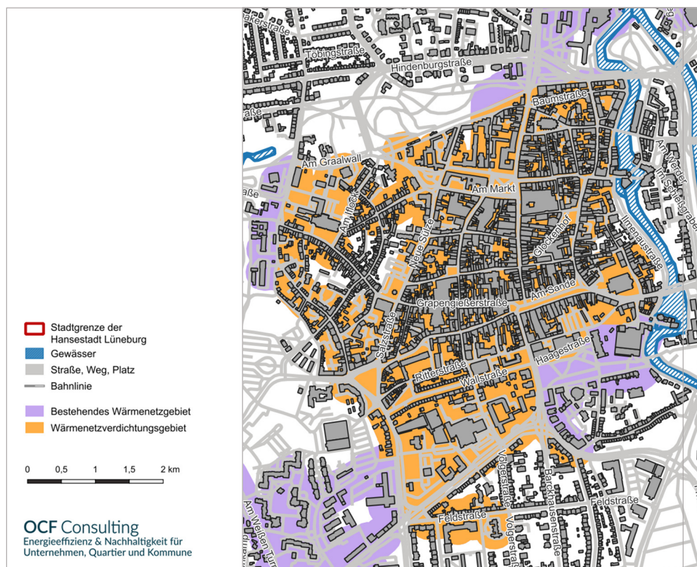
Abbildung 27: Wärmenetzverdichtungsgebiet innerhalb des Bestandswärmenetzes Mitte (violett) mit Nachverdichtungspotenzial (orange) (Quelle: OCF Consulting)
