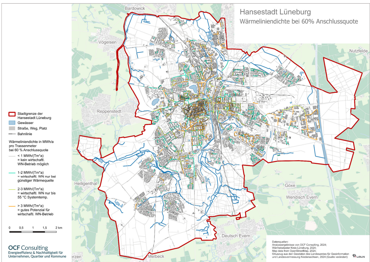
Abbildung 13: Wärmelinienichte Lüneburg für das Jahr 2022 in MWh pro Tm und Jahr bei 60 % Anschlussquote an ein fiktives Wärmenetz (WN) (Quelle: OCF Consulting auf Basis des Wärmekatasters Kreis Lüneburg)
